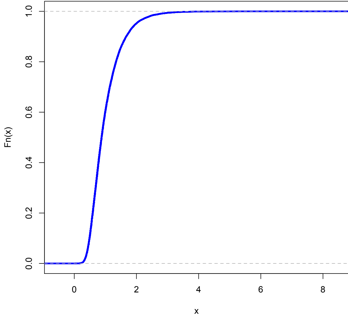
ecdf(nbarm)
